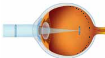
▲ La miopía se corrige con un lente biconcavo o divergente.
