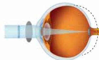
▲ La hipermetropía se corrige con un lente biconvexo o convergente.
